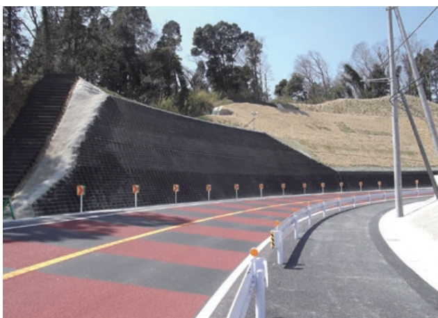
施主：東日本高速道路株式会社 工事名：首都圏中央連絡自動車道茂原北インターチェンジ工事 ■ 壁面勾配：1：0.5 ■ 壁高：6.75m ■ 壁面積：390㎡
