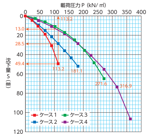
荷重—沈下曲線
