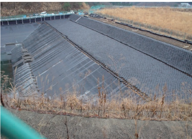
施主：三多摩地域廃棄物広域処分場組合 工事名：谷戸沢廃棄物広域処分場調整池補修工事 ■ のり面勾配：1：2.0 ■ 型式：T-100LP ■ のり面積：1,458㎡
