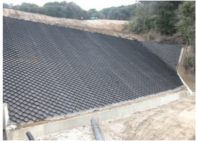
施主：九州地方整備局大隈河川国道事務所 工事名：東九州道(鹿屋～曾於)下高隈地区(第31区)改良工事 ■のり面勾配：1：1.8 ■型式：T-100LP ■のり面積：40,000㎡
