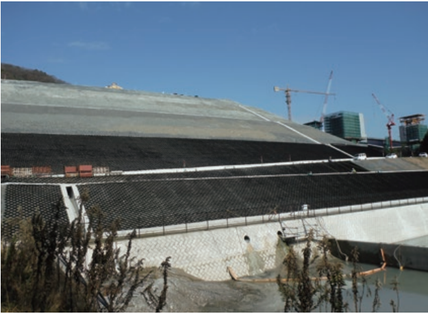
施主：西日本高速道路株式会社 工事名：新名神高速道路路面トンネル東工事 ■のり面勾配：1：1.8 ■型式：T-100LP ■のり面積：11,800㎡
