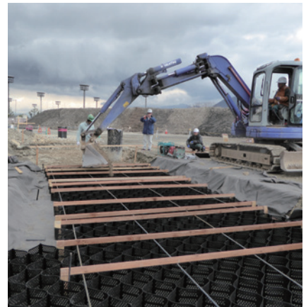
施主：山形県山形市役所 工事名：山形市新野球場建設建築工事 ■ 概要：T-150MP×2段
