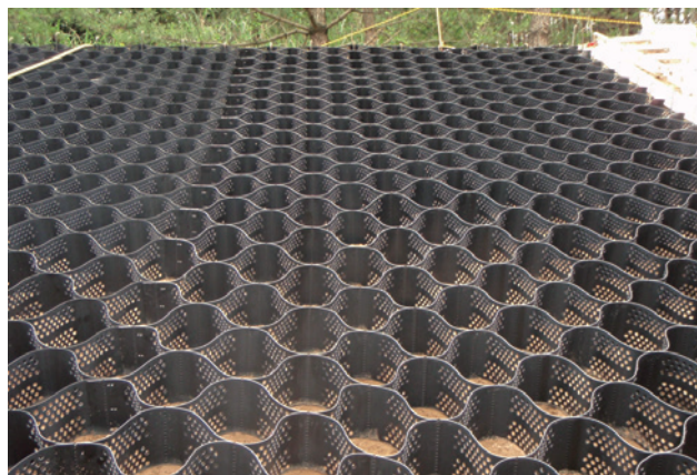
施主：東京電力株式会社 工事名：刈羽原子力発電所内のり面復旧工事 ■ のり面勾配：1：1.4、1.5 ■ 型式：T-150MP ■ のり面積：1,500㎡ ■ のり面勾配：1：1.6、1.7、1.8 ■ 型式：T-150LP ■ のり面積：700㎡
